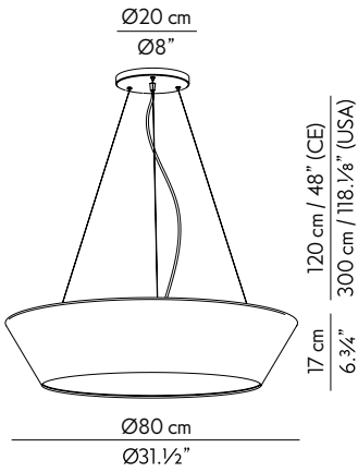
DA.S080.00 6 x E27 LED 12W
