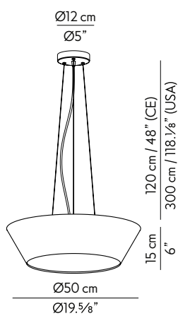
DA.S050.00 2 x E27 LED 12W
